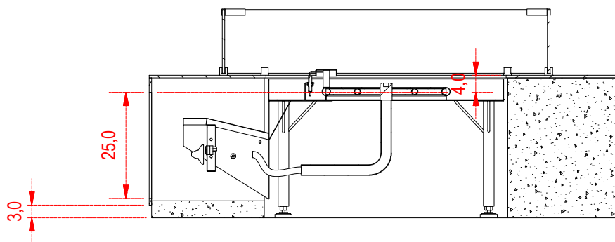
M-M (0,08 : 1)
