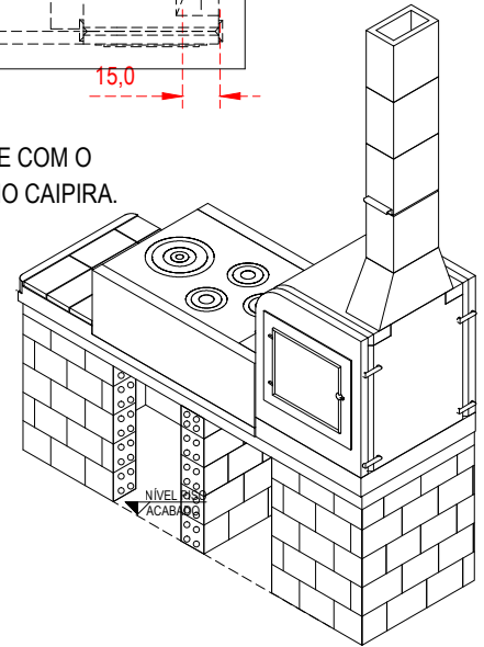
VISTA SUPERIOR DA EXECUÇÃO DA BASE
