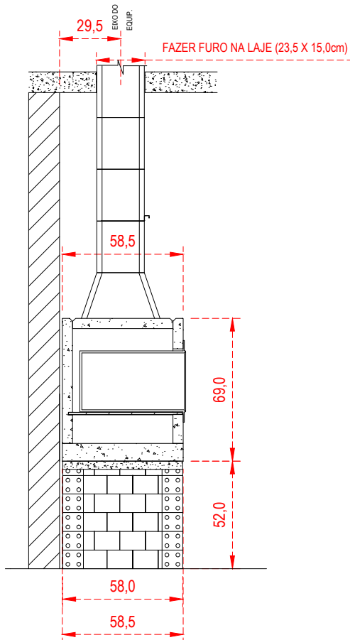
VISTA FRONTAL DA EXECUÇÃO DA BASE
