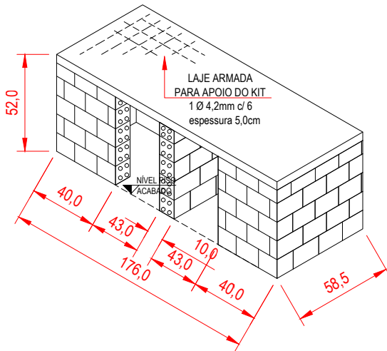
PERSPECTIVA DA BASE COM LAJE PARA KIT FOGÃO COM FORNO CAIPIRA.
