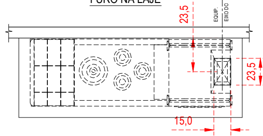
PERSPECTIVA DA BASE COM O KIT FOGÃO COM FORNO CAIPIRA.
