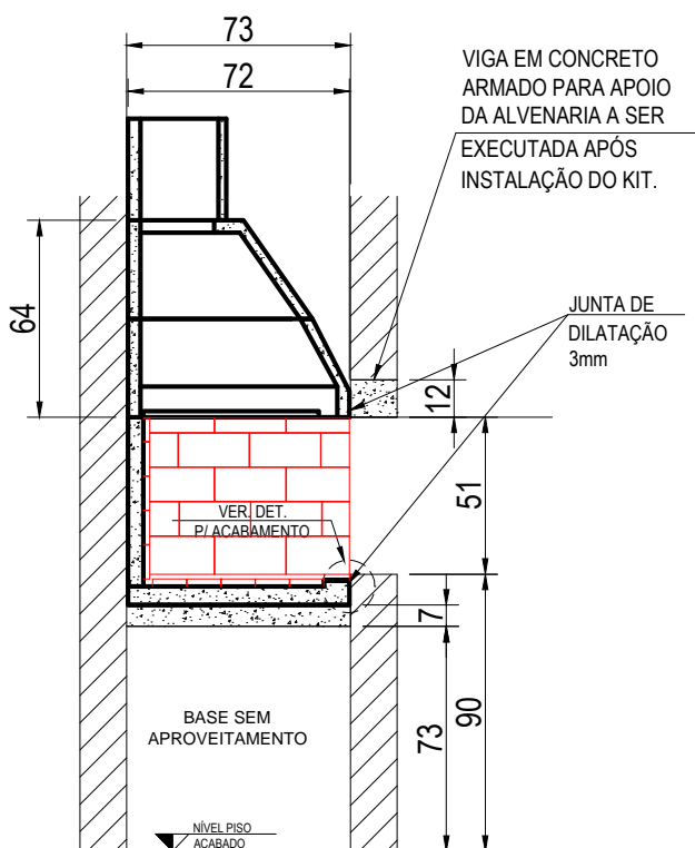
CORTE COM ALVENARIA DE FECHAMENTO A SER EXECUTADA APÓS INSTALAÇÃO DO KIT.
