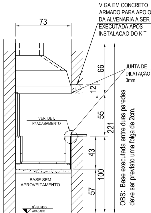
CORTE COM ALVENARIA DE FECHAMENTO A SER EXECUTADA APOS INSTALACAO DO KIT.
