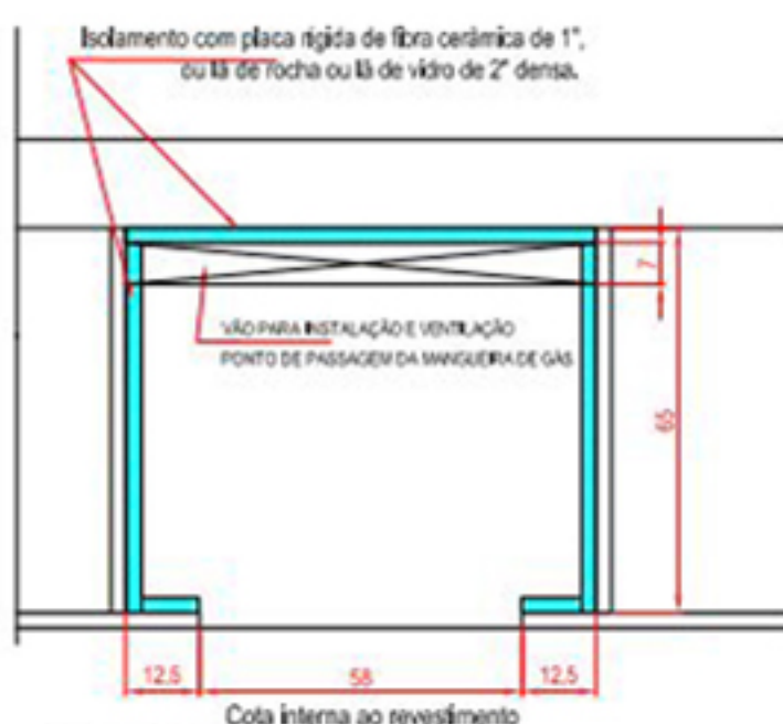
VISTA SUPERIOR
