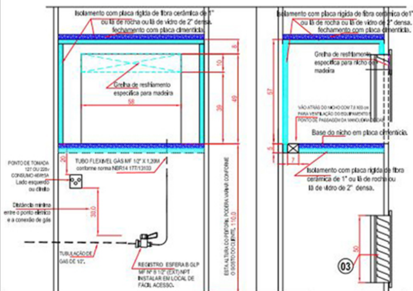
VISTA LATERAL
